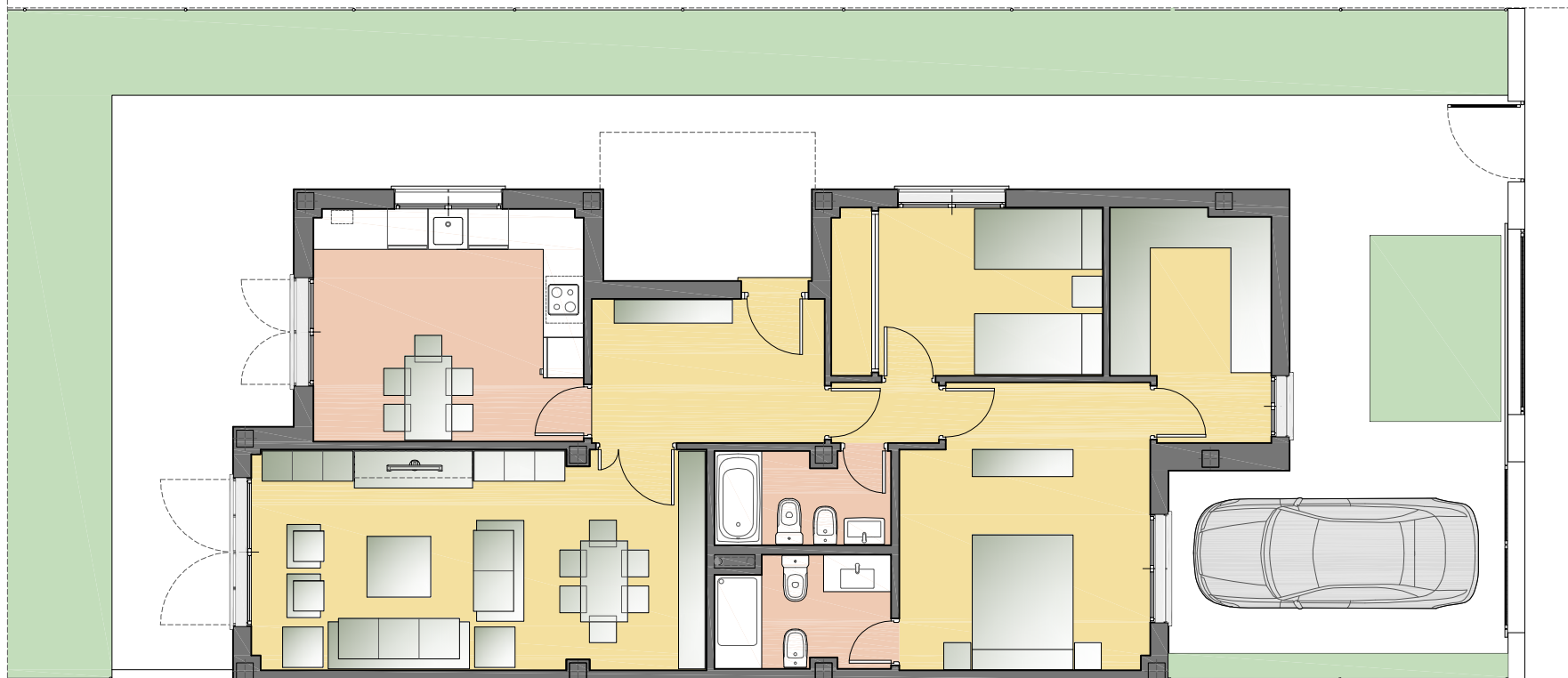
PLANO DE PLANTA. ESCALA 1:100.
